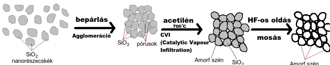
A mezopórusos szén feltételezett képződési mechanizmusa
