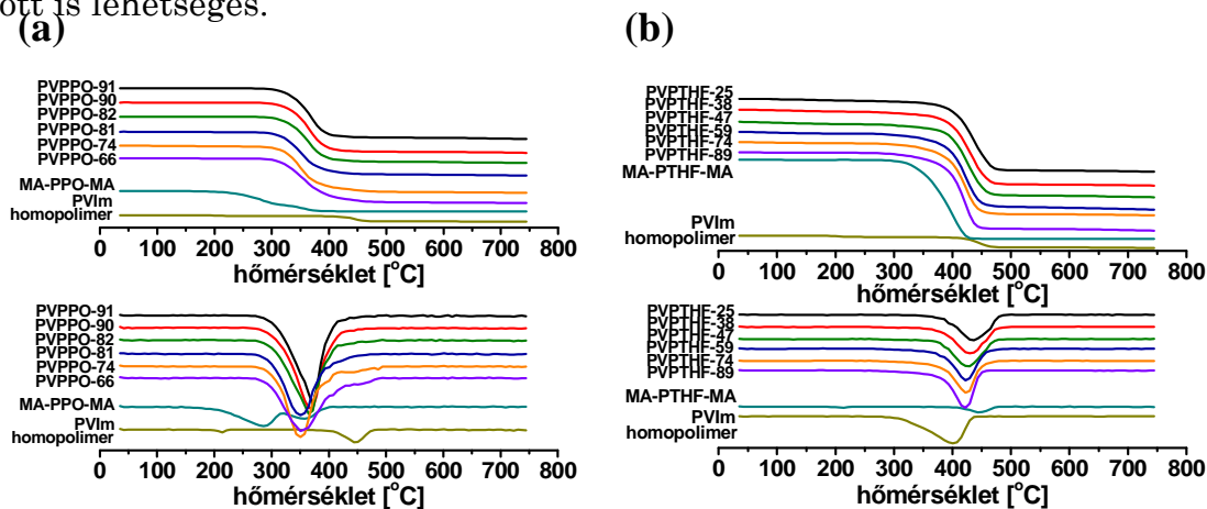
16. ábra: Termogravimetrikus (TG) és derivatív termogravimetrikus (DTG) görbék; (a) PVIm- l -PPO AKT sorozatra és (b) PVIm- l -PTHF AKT sorozatra
