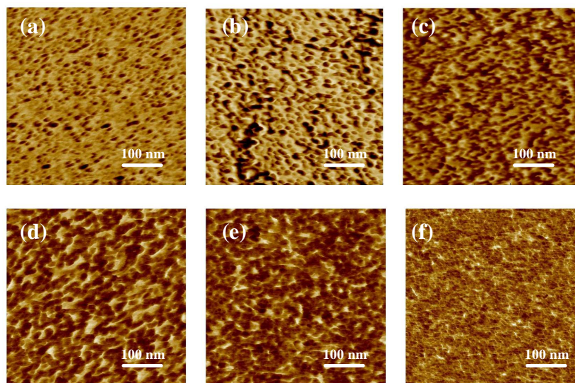
18. ábra: AFM képek PVIm- l -PTHF AKT sorozatról (500 nm x 500 nm) (a) P2-25 (25 wt% PTHF); (b) P2-38 (38 wt% PTHF); (c) P2-47 (47 wt% PTHF); (d) P2-59 (59 wt% PTHF); (e) P2-74 (74 wt% PTHF); (f) P2-89 (89 wt% PTHF); (a rugalmas PTHF fázis sötétbarna, a kemény PVIm fázis világosbarna színű)
