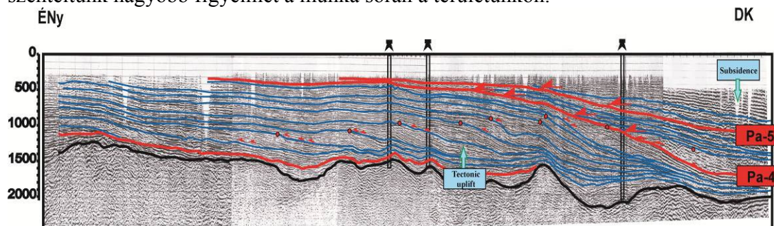
2. ábra Szekvencia sztratigráfiai értelmezés egy ÉNY-DK-i irányú regionális szelvény mentén a vizsgált kutatási terület központi részén, a kanyonóvtól K-re.
