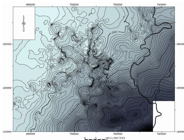
9. ábra A Pa-4 szekvenciahatár mélységtérképe, valamint az Alpár kanyonrendszer mai morfológiája (Juhász et al. 2007, in rev.). Jól látható, hogy az árokrendszer a Makói-árok irányában lejt.
