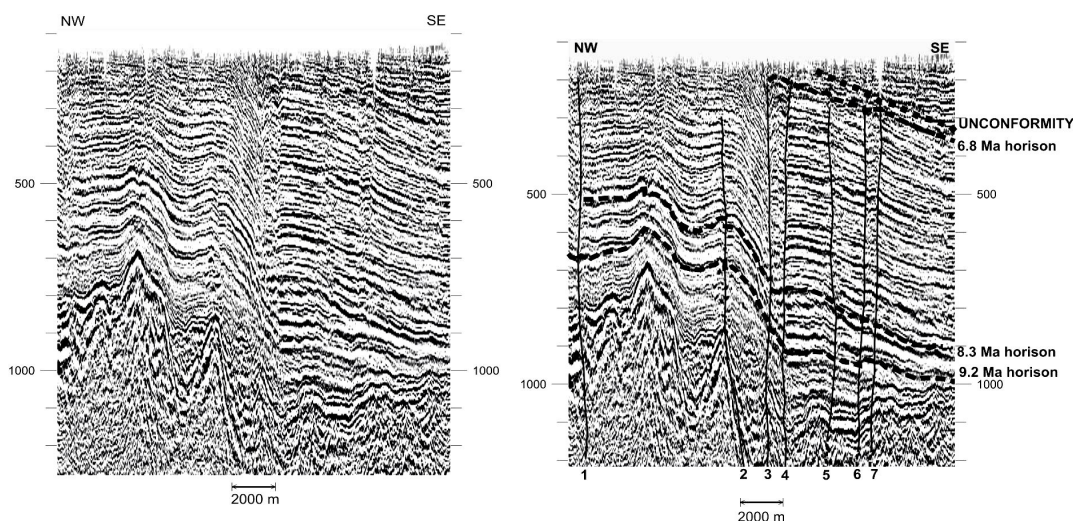
8. ábra ÉNY-DK irányú szeizmikus szelvény értelmezett és értelmezelen változatban. A szelvény nyomvonala az 7. ábrán látható. A szelvényen korrelált 9.2, 8.3, 6.8 millió éves szeizmikus horizontok korának meghatározásánál a Kaskantyú-2 végig magvétel MAFI alapfúrás és a Kiskunhalas Nyugat 3 fúrások magnetosztatográfiai és radiometrikus (K/Ar) koradataira támaszkodtunk. A Kaskantyú-2 fúrásban harántolt miocén végi diszkordancia Juhász et al (1997) szerint 6.2 és 3.9 millió év közötti hiátust reprezentál a Kask-2 fúrás térségében. A szeizmikus szelvényen látható, a miocén képződményeket felülről határoló diszkordanciát, úgy tűnik nem vetik el a #5, #6, #7 jelű vetők. A #3, #4 jelű oldaleltolódás minden bizonnyal még a kvarterben is aktív volt. A #2 jelű vető szemmel láthatóan átmetszi (azaz annál fiatalabb) a térrövidüléshez kapcsolódó redőt.
