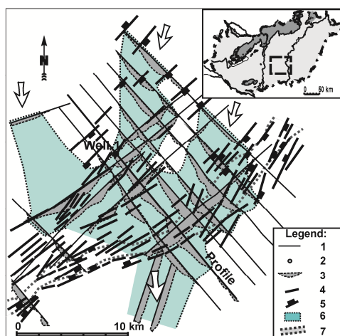
6. ábra. A kanyon rendszer területi elterjedése és hálódigramja, valamint a terület tektonikai értelmezése (Juhász et al. 2007, in rev.). Legend: 1. sz. eismikus háló, 2. fúrás, 3. kanyon, 4. normal vető, 5. Riedel-vető, 6. kanyon ágak, 7. gyökérszóna
