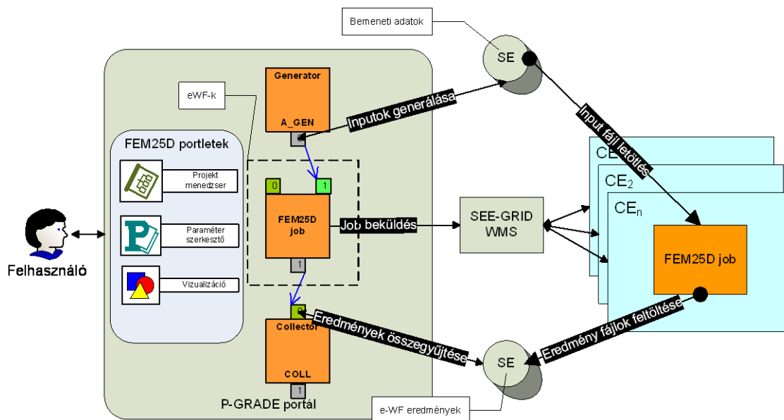
11. ábra GRID alkalmazás struktúrája a 2.5D FEM modellező rendszer esetén
